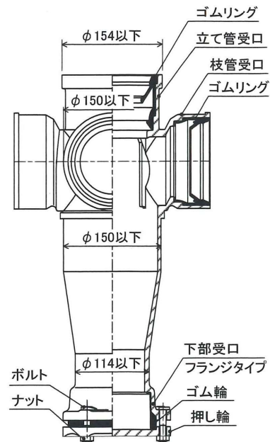
(イ) フランジタイプ（受口）
